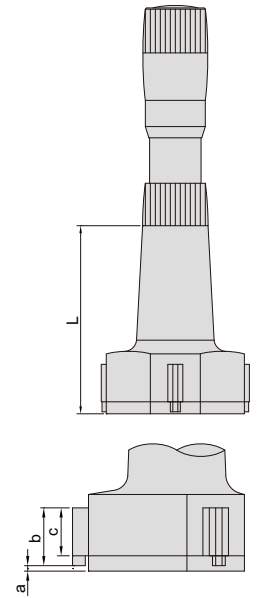
C型 50-300mm, 三点式 硬质合金测量面
