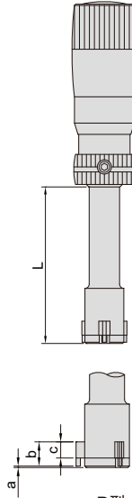
B型 12.5-50mm, 三点式 硬质合金测量面
